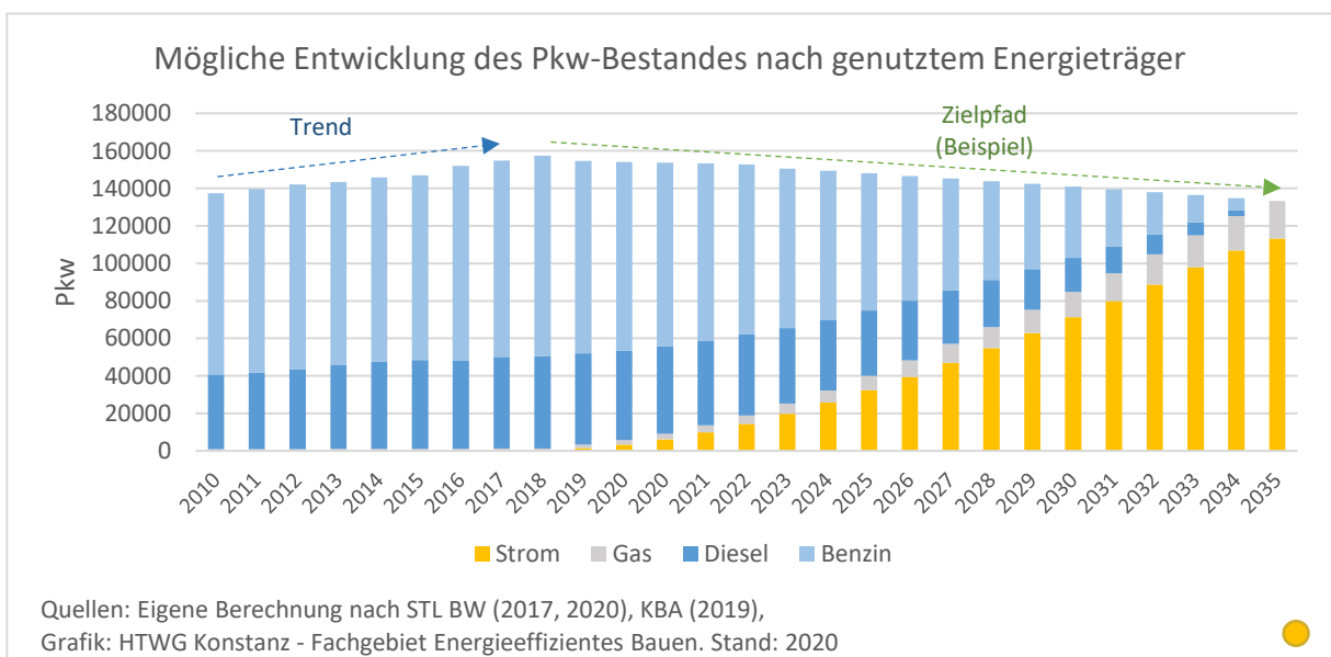
Abbildung 117: Mögliche Entwicklung des Pkw-Bestandes im Klimaschutzscenario 2
